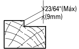
Fig. 2-C (Ranurado)
