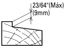
Fig. 2-D (Ahusamiento)
