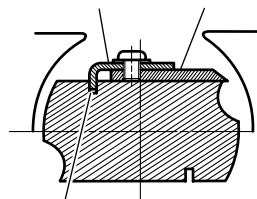
Fig. 10 (Installation correcte)
