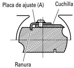
Fig. 10 (Instalación correcta)
