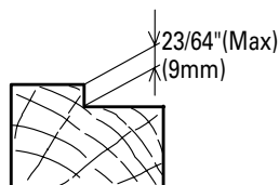
Fig. 2-C (Feuillure)
